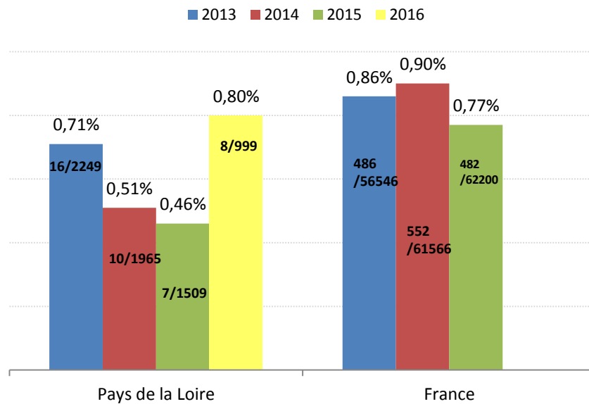
Taux de TRODs positifs parmi les TRODs réalisés par les structures associatives
